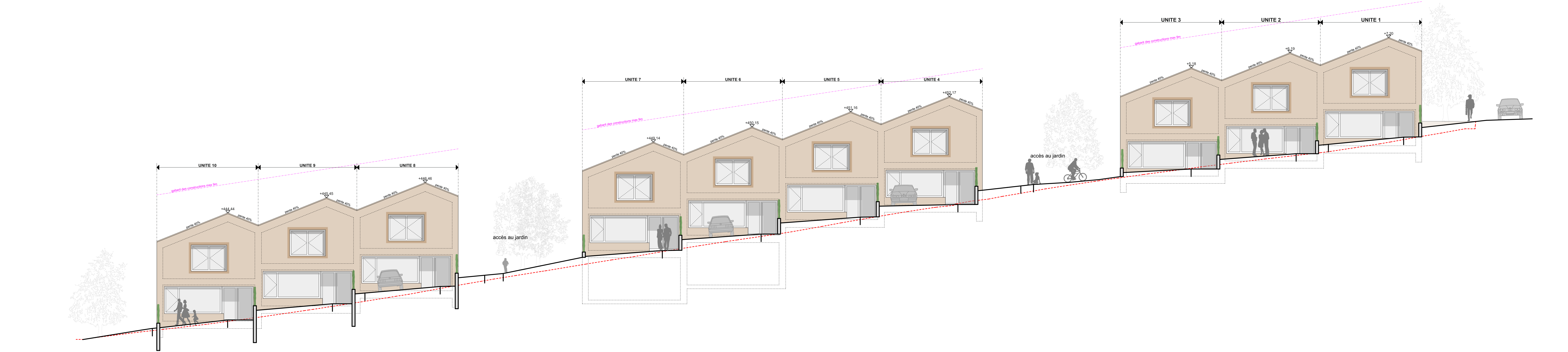
ELEVATION NORD
